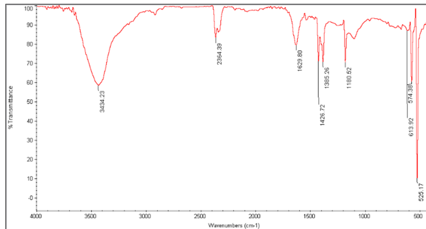
شکل ۲: طیف سنجی FT-IR هیدروکسیل فولرن
