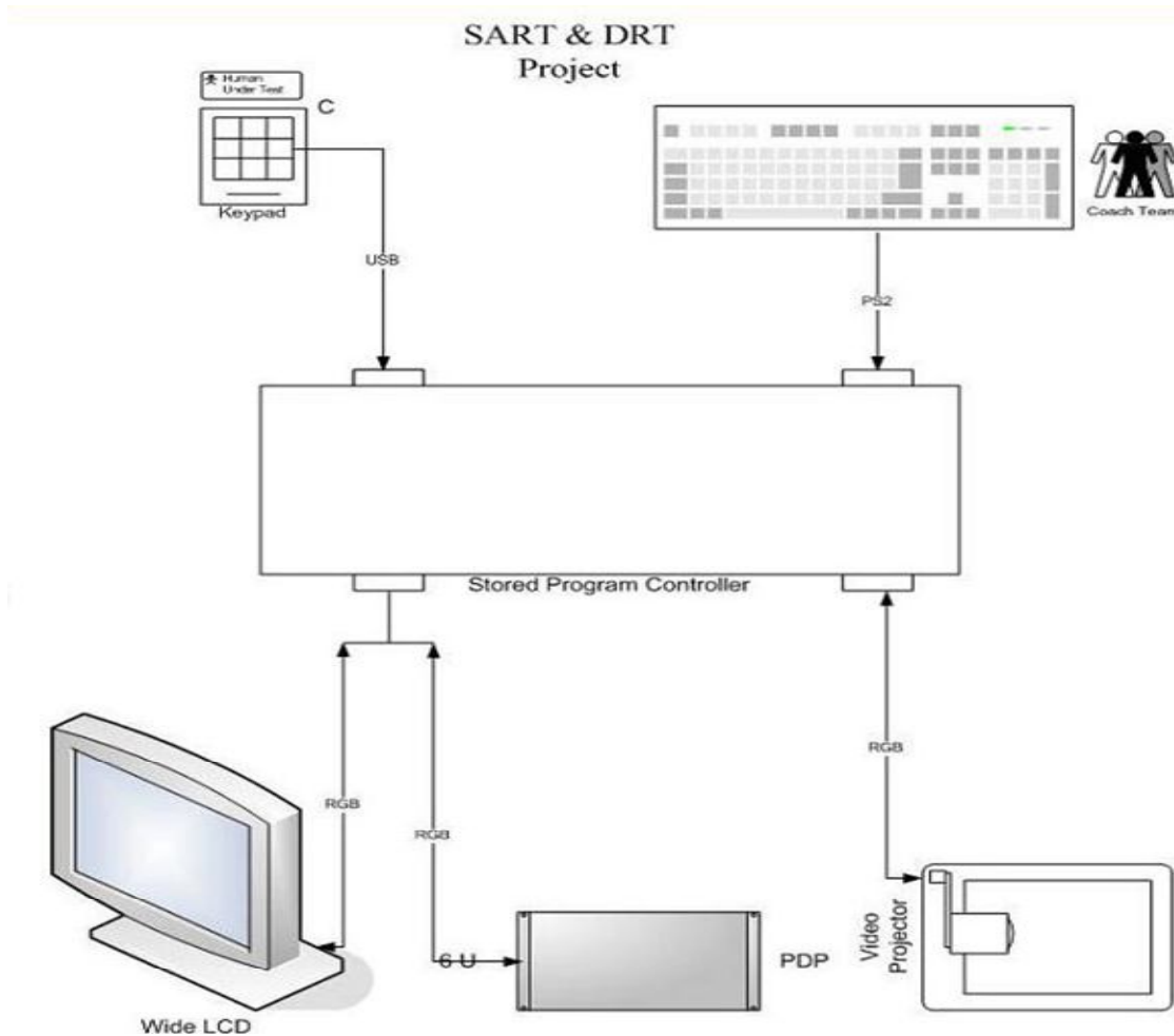
شکل 1- نمایش اجزای مختلف سامانه
