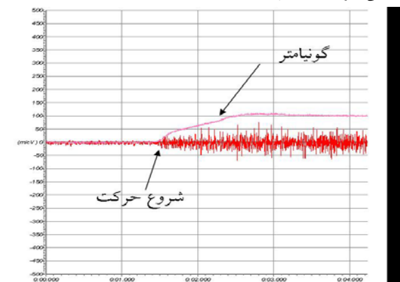
شکل ۱: نمونه‌ای از سیگنال الکترومیوگرافی و نحوه جابجایی گونیامتر الکتريکال
