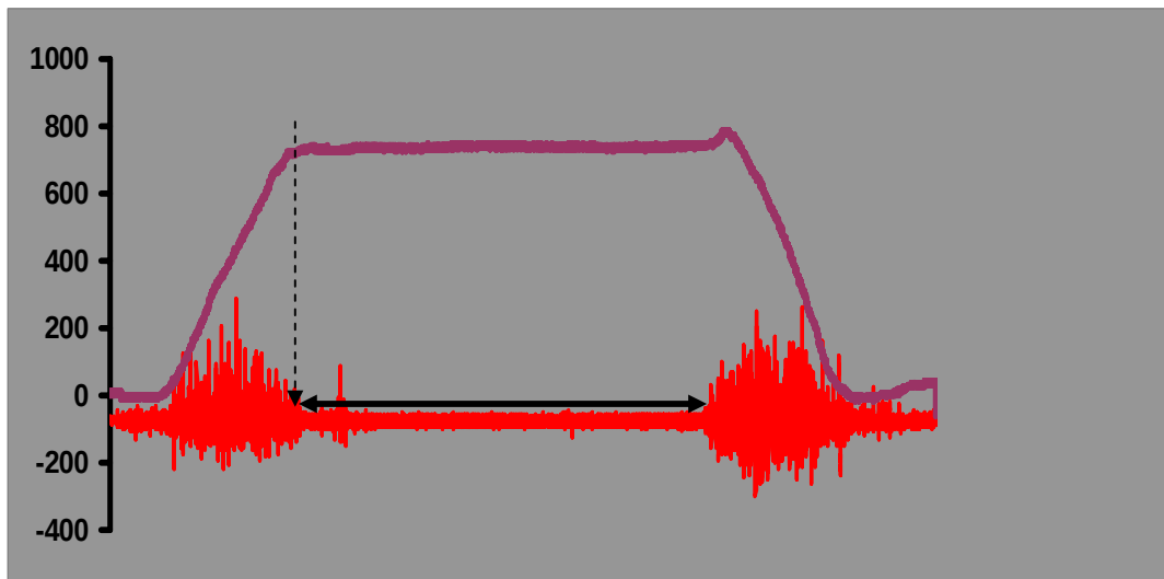
شکل ۱ - قسمت بالا مراحل مختلف تست فلکشن-اکستنشن را نشان می دهد قسمت پایین سیگنال الکترومیوگرافی و منحنی مربوط به گونیامتر دیجیتال و دوره سکوت میوالکتریک را نشان می دهد.
