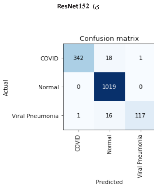
شکل ۳: تفسیر نتایج به دست آمده از مدل‌های مختلف به کار گرفته شده در قالب ماتریس درهم‌ریختگی
