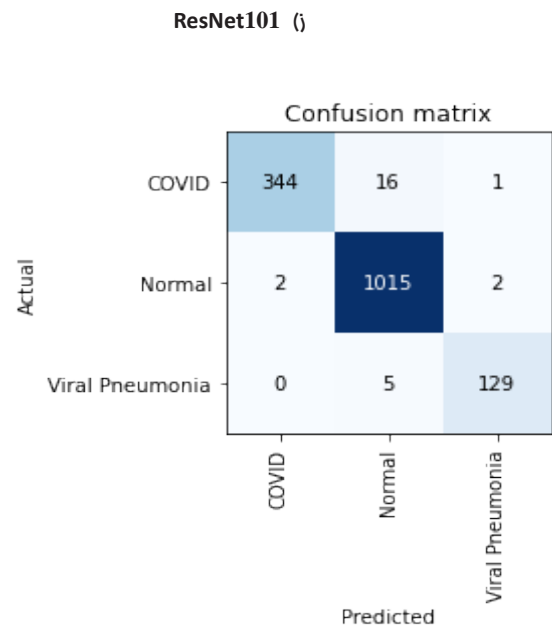
شکل ۳: تفسیر نتایج به دست آمده از مدل‌های مختلف به کار گرفته شده در قالب ماتریس درهم‌ریختگی
