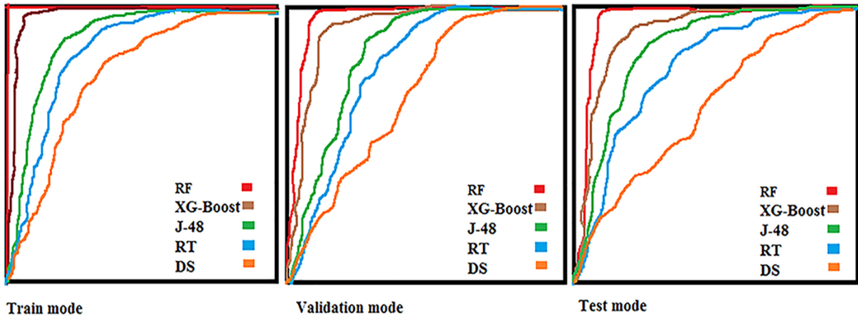
شکل ۱: سطح زیرمنحنی فصوحیت گیرنده عامل مدل‌های منتخب
