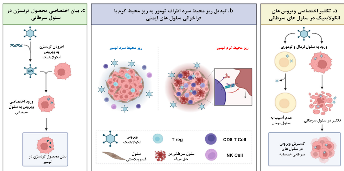
شکل ۱: نمای کلی از نمونه‌ی عملکرد ویروس‌های انکولایتیک
