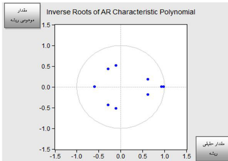
نمودار \lambda معکوس ریشه‌های مشغله‌ی AR های
