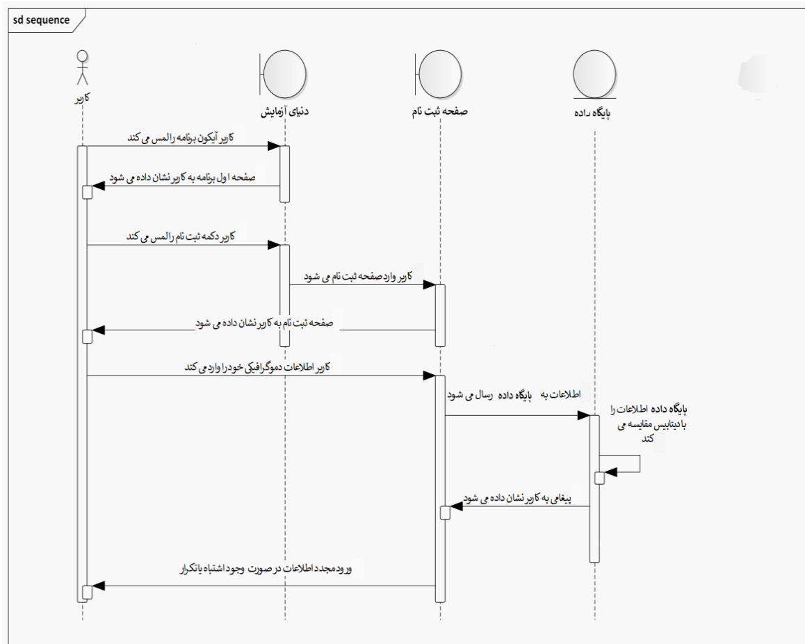
شکل ۲: نمودار توالی ثبت نام و امراز هویت
