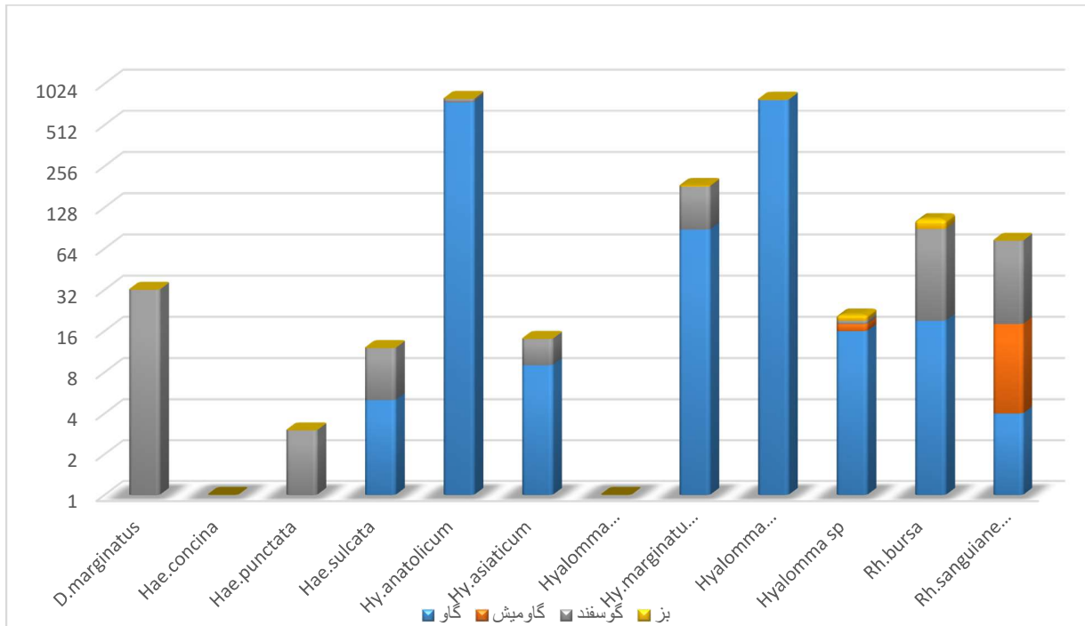
نمودار ۱- فراوانی کنه‌های سخت صید شده به تفکیک گونه در شهرستان های اهر و کلیبر استان آذربایجان شرقی، سال ۹۷-۱۳۹۶
