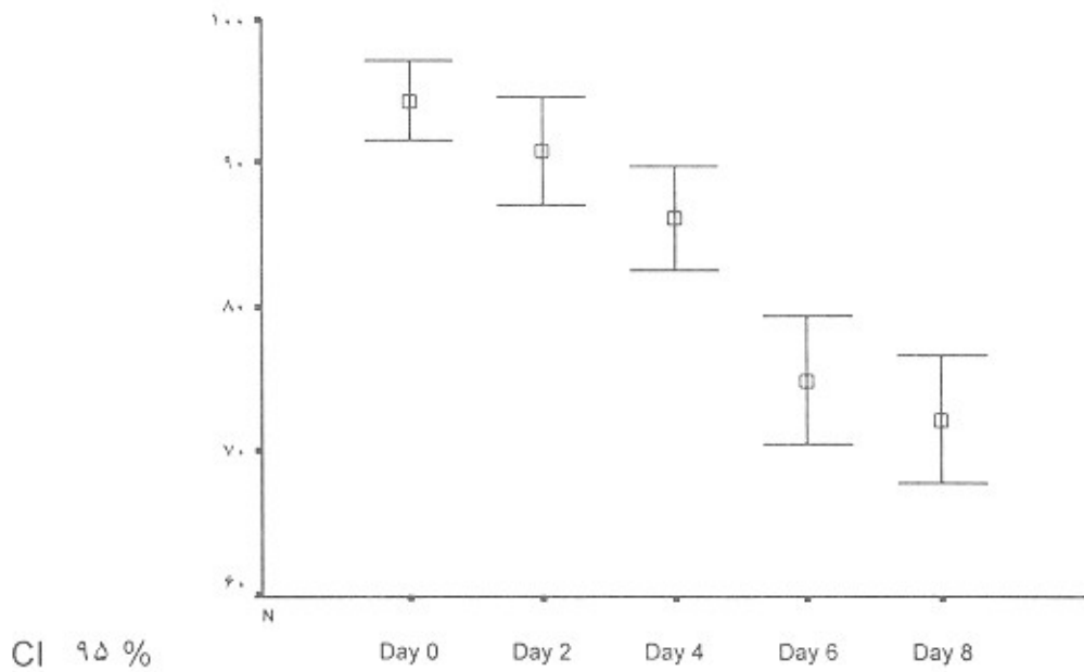
نمودار ۳- سیر تغییرات درصد زنده ماندن سلول‌ها بعد از جداسازی سلول‌های تک هسته‌ای نمونه‌های خون محیطی موبیلیزه نگهداری شده در دمای 4°C تا هشت روز
