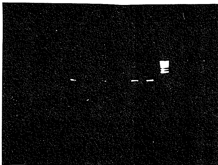
شکل شماره ۱- ژل الکتروفورز شده حاوی باندهای ۲۰۲ تکثیر شده ژل mec A به همراه DNA Marker
