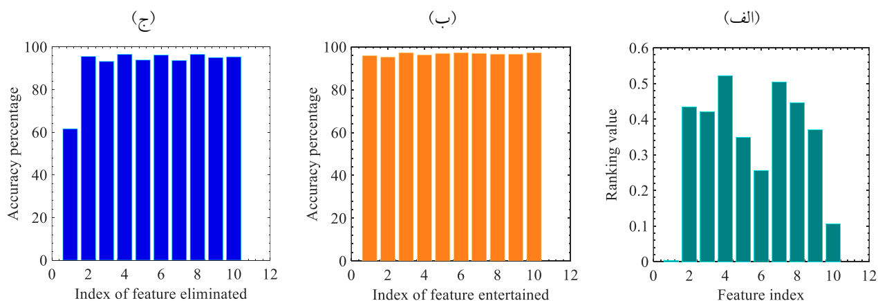
شکل ۳- (الف) رتبه‌بندی حاصل از اطلاعات متقابل به‌نحار شده به‌ازای همه ویژگی‌های موجود در مجموعه داده سرطان پستان. (ب) دقت محاسبه شده به‌ازای هر ویژگی اضافه‌شده به مجموعه ویژگی‌های انتخابی در رویکرد شمول ویژگی. (ج) دقت به‌دست آمده از حذف ویژگی با پایین‌ترین رتبه در روش خروج ویژگی.
