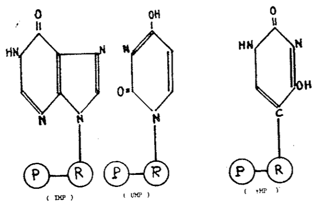
شماي شماره ۳ - فرمول ساختمانی اوریدین منوفسفات کاذب ،
