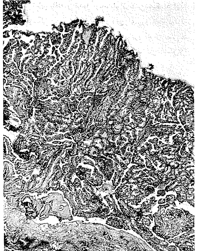
شکل ۲- کارسینوم پاپیلر مجرای تیروگلوبوس- بافت تومورال پاپیلر که در در داخل خنجره‌ای قرار دارد- جدار خنجره را یک ردیف سلولهای مکعبی منبسط کرده است. بد کالکوسفریت و کالکونهای آهکی شده توجه شود
