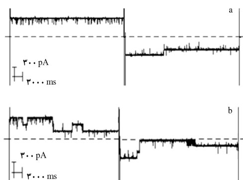
شکل ۲: جریان عبوری از کانال منفرد OmpF در ولتاژ \pm 140 میلی‌ولت، در دمای 20^{\circ}\text{C} و \text{pH } 7/4 به مدت ۱۰ دقیقه در دو حالت (a) حالت کنترل (وضعیت خاموش گوشی تلفن همراه) (b) تحت تابش امواج گوشی تلفن همراه (وضعیت روشن گوشی)
