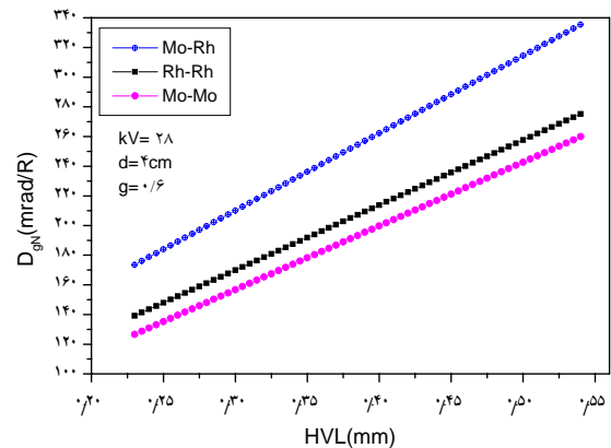
شکل-۳: تغییرات متوسط دوز جذبی غده‌ای بر حسب HVL اشعه X دستگاه ماموگرام برای سه آرایش هدف - فیلتر و به ازای kV=28 , d=4 cm و G=0.6
