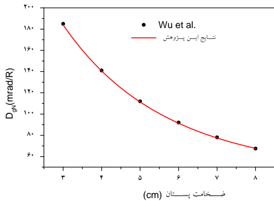
شکل-۴: نتایج مونت کارلوی Wu و همکارانش و نتایج حاصل از کد به ازای ضخامت پستان (cm) و D_{gH} (mrad/R). d=4 cm, HVL=0.26 mm و G=0.5
