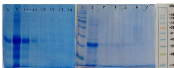
شکل ۳: نتیجه تخلیص به‌وسیله ستون کروماتوگرافی نیکل
