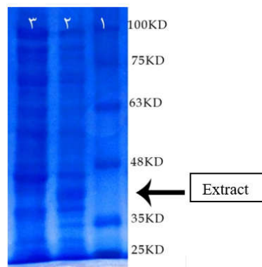
شکل ۱: نتیجه SDS-PAGE پروتئین همگلوتینین ۱ (HA1) پس از تخلیص
