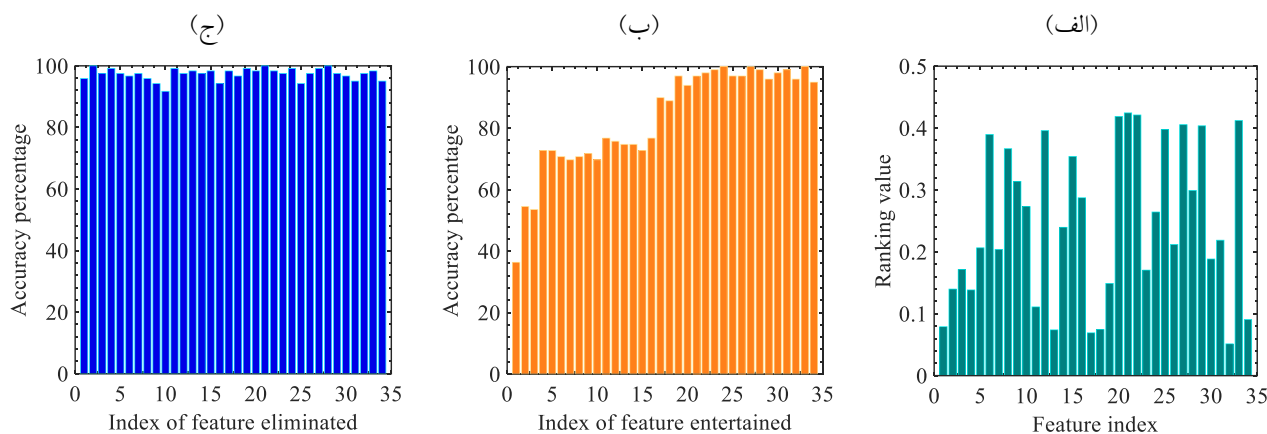
شکل ۱۱: (الف) رتبه‌بندی حاصل از اطلاعات متقابل بهنجار شده به‌ازای همه ویژگی‌های موجود در مجموعه داده پوست‌شناسی. (ب) دقت محاسبه شده به‌ازای هر ویژگی اضافه‌شده به مجموعه ویژگی‌های انتخابی در روش شمول ویژگی. (ج) دقت به‌دست آمده از حذف ویژگی با کمترین رتبه در روش خروج ویژگی.
