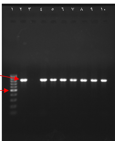
شکل- ۲: نتیجه آزمون PCR ژن blaVIM-1 (طول محصول: PCR ۸۰۱ bp). ۱- DNA Ladder، ۲- Positive Control، ۳- Negative Control، ۴- نمونه ۱۰-۴
