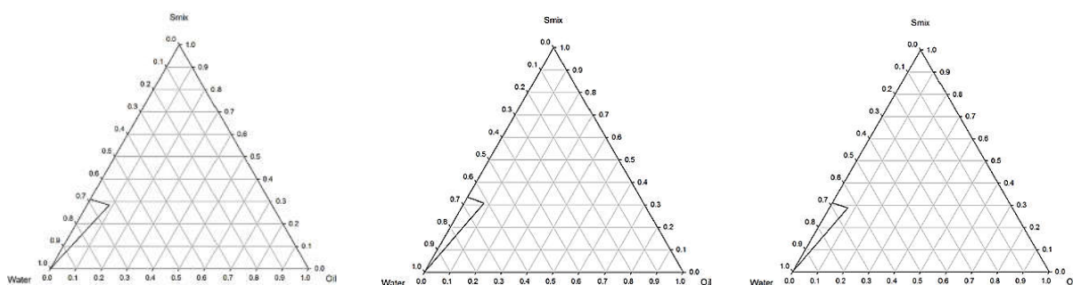
شکل ۱: نمودارهای شبه‌سه‌فازی (الف) نسبت توپین ۸۰ به ۸۰ اسپن ۸۰:۱ = (ب) نسبت توپین ۸۰ به ۸۰ اسپن ۹۰:۱ = (ج) نسبت توپین ۸۰ به ۸۰ اسپن ۱۰:۱ =
